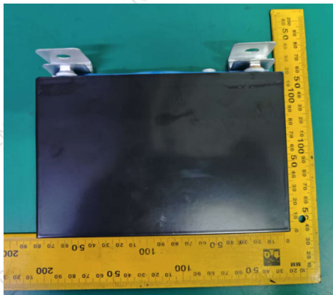
电芯 Cell
